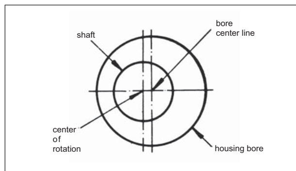
Fig.6- Shaft Offset
